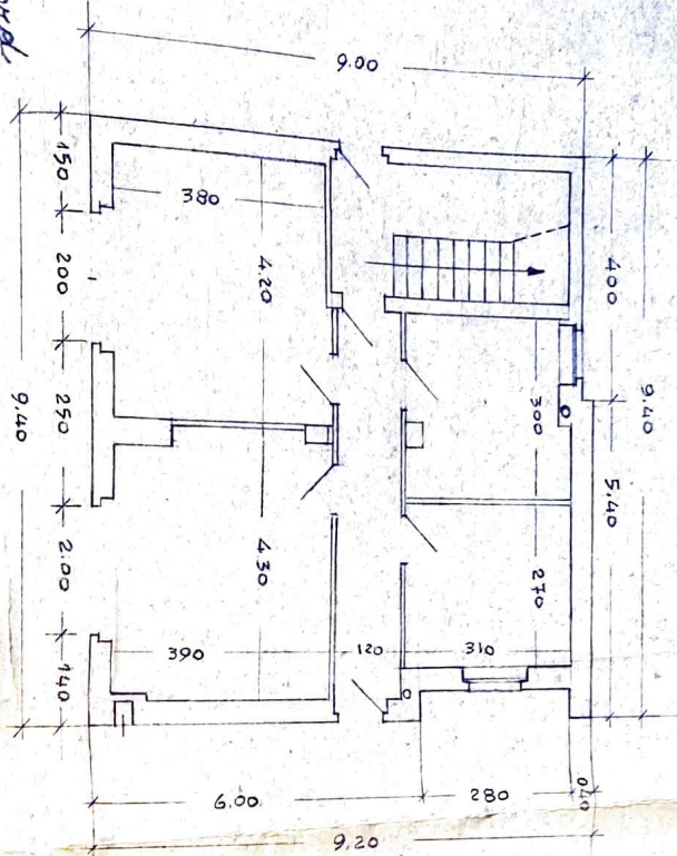
PIANTA PIANO CANTINATO
