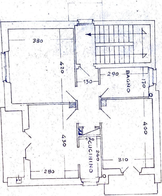
PIANTA PIANI I e II
